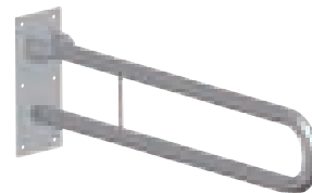
Sklopné držadlo k WC Ø 30 mm, vr. montážnej sady dĺžka (rozteč): 700 mm, celková dĺžka: 715 mm č. L2161005 (195,00 € / 5.875 Sk)
