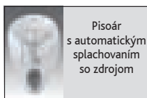
Pisoár NOVA (Felix) s radarovým splachovačom s int. zdrojom č. 2607RZ (447,00 € / 13.466 Sk), skladajúci sa z: pisoár č. 26000, radarový splachovač pre napájanie z el. siete 230V AC, odpadový sifón 1L, montážna sada
