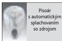
Pisoár NOVA TOP (Alex) s radarovým splachovačom s int. zdrojom, č. 6618RZ (475,00 € / 14.310 Sk) skladajúci sa z: pisoár č. 066000, radarový splachovač pre napájanie z el. siete 230V AC, odpadový sifón 1L, montážna sada
