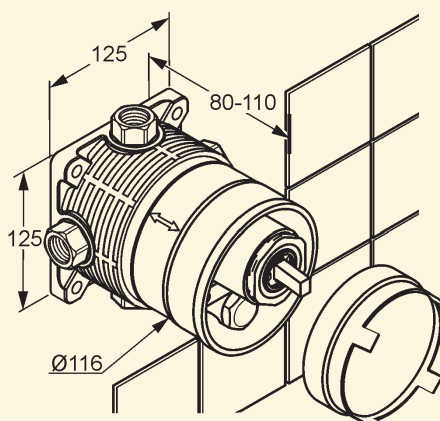
Flexx.Boxx: inštalačné rozmery.
